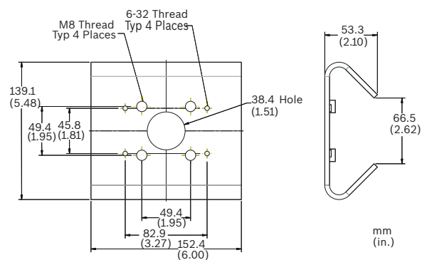
LTC 9213/01 Размеры адаптера для установки на столб
