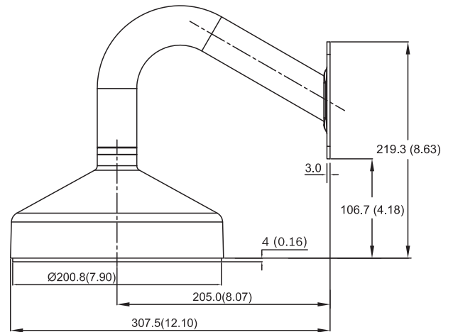
VDA-832FHD-WMT dimensioni installazione a parete
