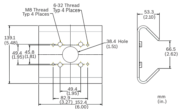
LTC 9213/00 dimensioni adattatore per installazione su palo
