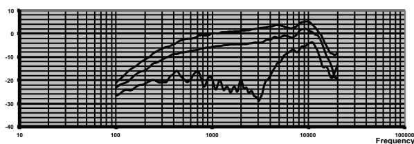
頻率響應 (開啟角度: 0、90 和 180 度)
