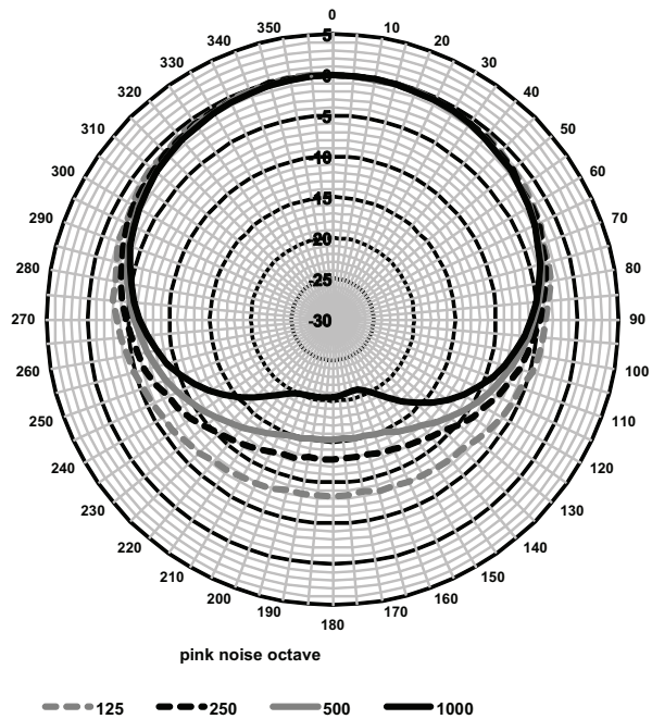
極座標圖 (以粉紅噪訊衡量)
