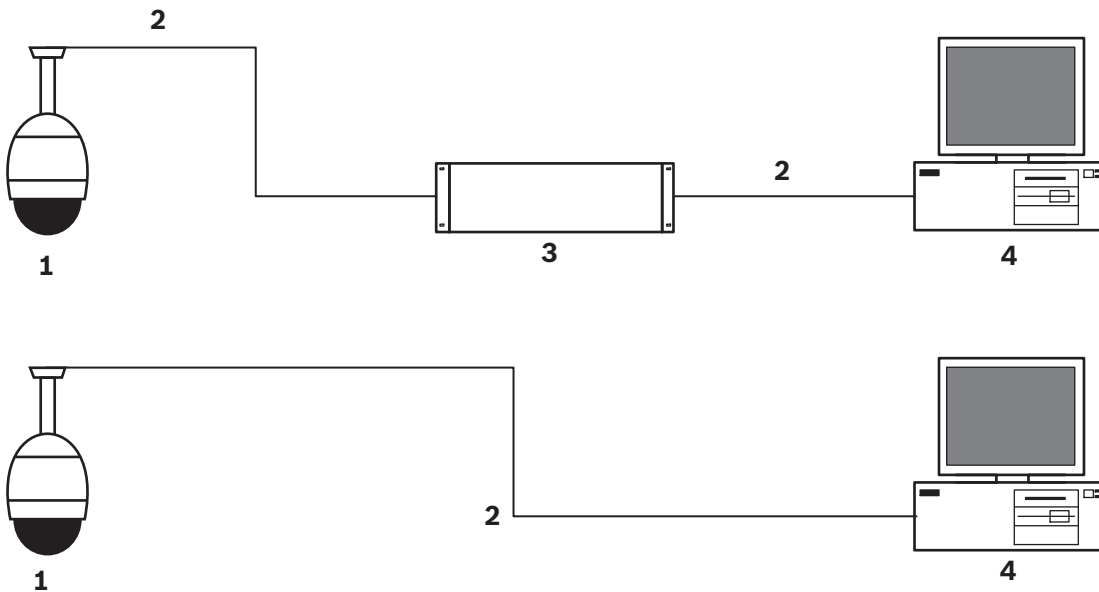
Figura 8.1: Configuración del sistema de la AUTODOME IP
