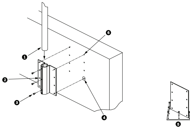
Figura 7.1: Soporte de sujeción en pared y placa de montaje en azotea
