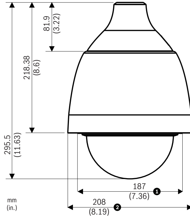
Figura 7.1: Dimensiones de AUTODOME 5000 para interiores/exteriores
