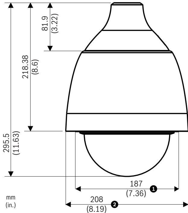
AUTODOME 5000 尺寸
