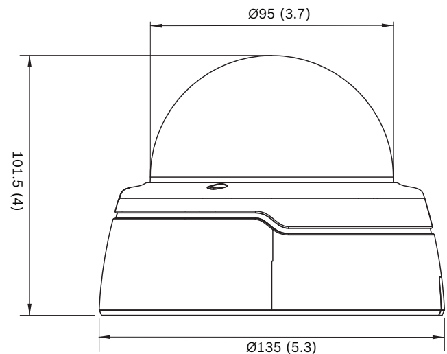
Размеры (мм/дюймы)
