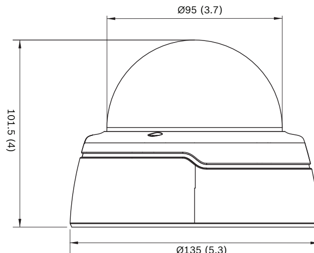
Dimensioni (mm/pollici)
