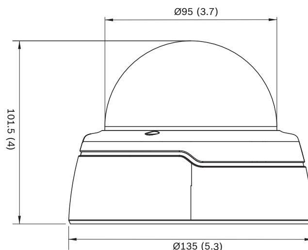
Dimensioni (mm/pollici)
