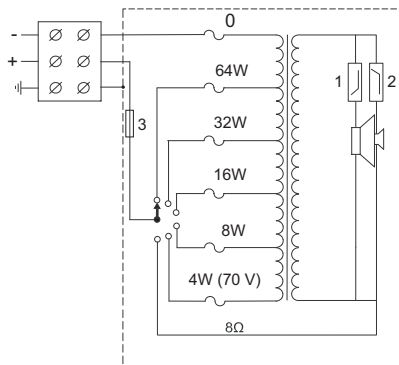
Sơ đồ nối mạch (1: Bộ Lọc Tần Số Thấp, 2: Bộ Lọc Tần Số Cao, 3: Cầu chì nhiệt)
