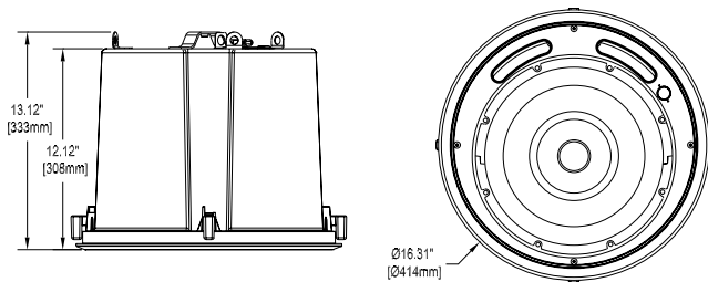
Kích thước tính theo Inch / [mm]
