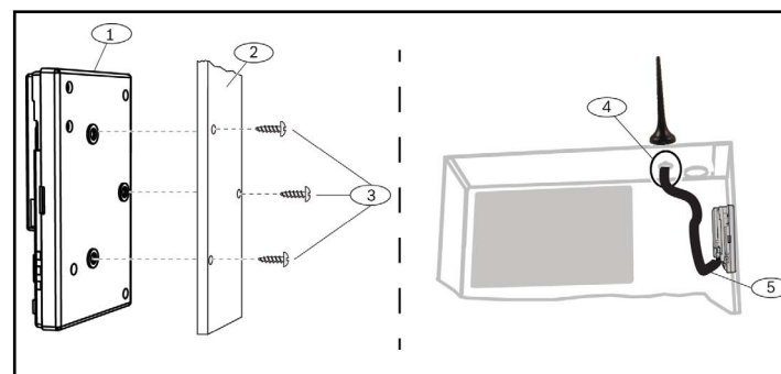
Figure 3.3 : Installation du module
