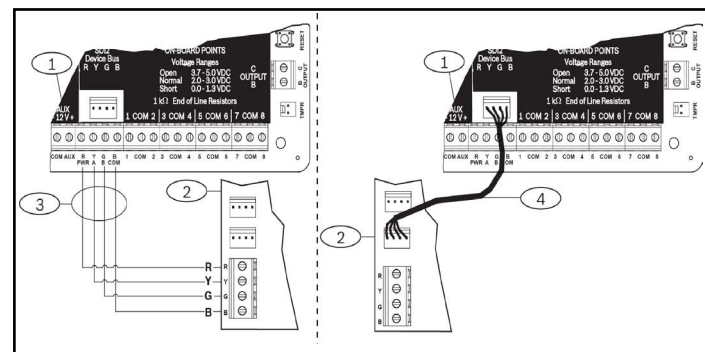
Figure 3.3 : Utilisation de la barrette de connexion SDI2 ou de câble d'interconnexion SDI2 (centrale B5512 illustrée).
