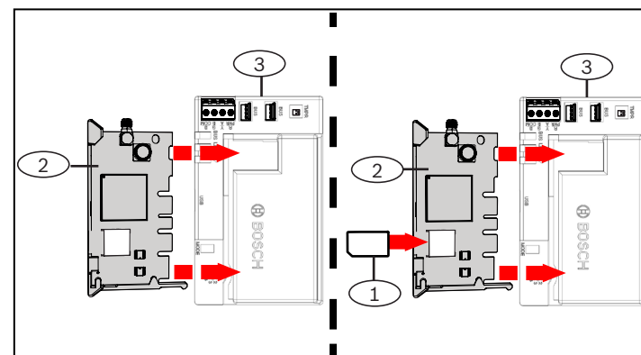
Figure 3.1.2 : Insertion du module de communication
