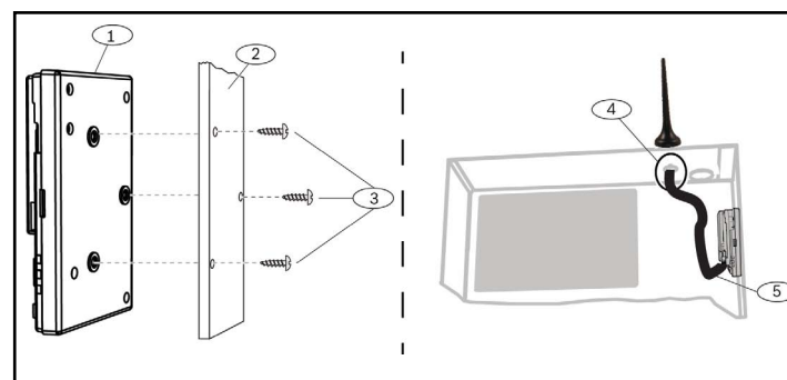
Figura 3.3: Instalación del módulo
