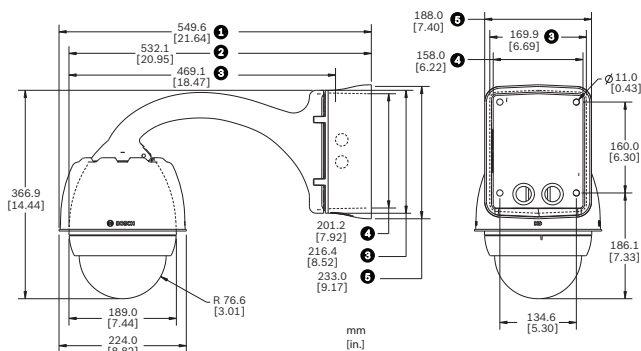
Dimensioni AUTODOME 7000: pendente, tubo
