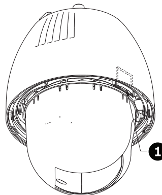
Камера серии AUTODOME 7000: разъем для карты SD
