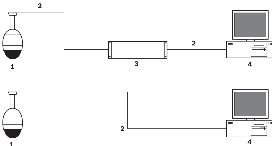
Figure 9.1: Configuration du système AUTODOME IP
