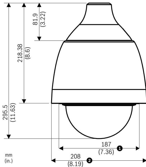
Afbeelding 7.1: Afmetingen AUTODOME 5000 binnenshuis/buitenshuis
